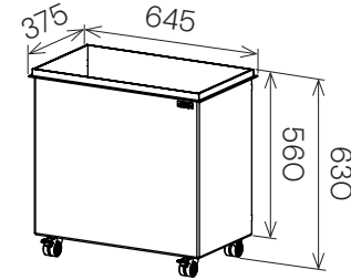
RIM 645w x 375d x 630h
